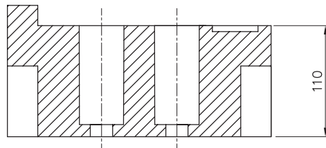
DOORSNEDE A-A scale 2:1
